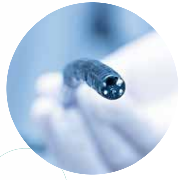
小さな内視鏡の先端部には、ライト、対物レンズ、送気・送水ノズル、吸引口/鉗子口が集まる
